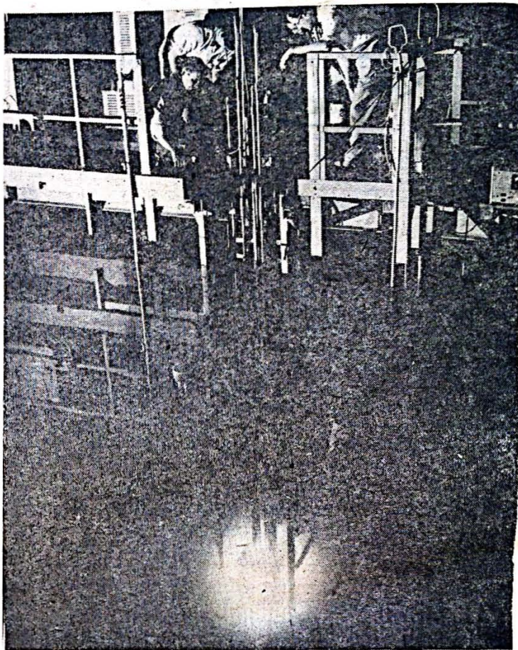
El interior del reactor tipo piscina en operación. (Foto izquierda).
